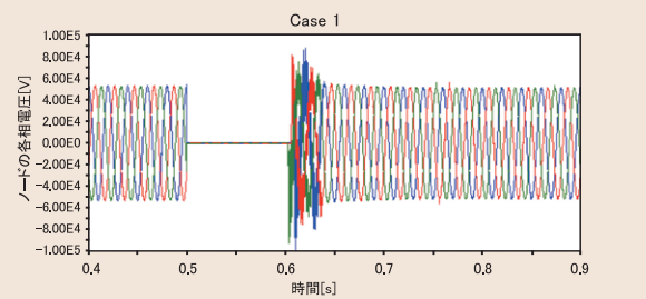
図2 XTAPを用いたSTATCOMの電圧制御特性(解析例)
