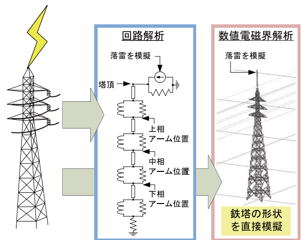
図4-1 雷サージ解析のための鉄塔モデル
