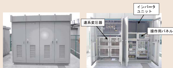
図3 既開発STATCOM(据置型)
