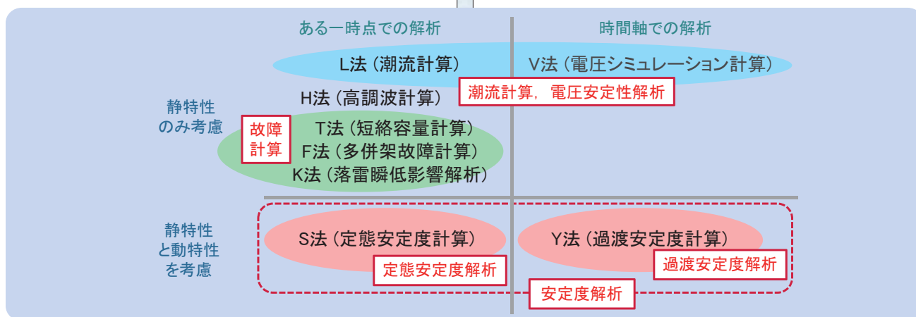
図2-1 CPATを構成するプログラム
